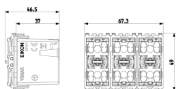
Zeichnung Dimensionen
