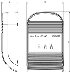
Zeichnung Dimensionen
