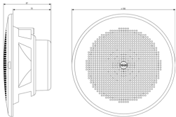
Zeichnung Dimensionen
