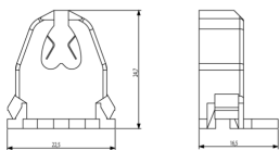
Zeichnung Dimensionen
