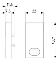
Zeichnung Dimensionen
