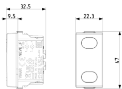
Zeichnung Dimensionen
