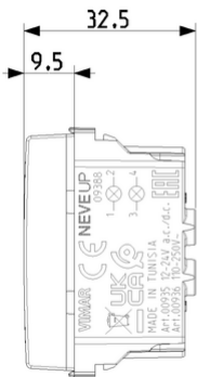
Zeichnung Dimensionen
