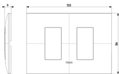
Zeichnung Dimensionen
