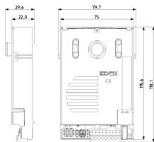
Zeichnung Dimensionen
