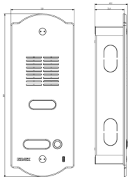
Zeichnung Dimensionen
