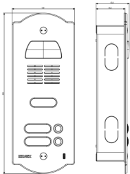
Zeichnung Dimensionen
