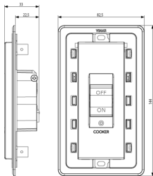
Zeichnung Dimensionen
