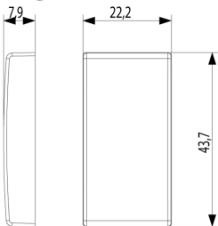
Zeichnung Dimensionen
