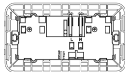
Zeichnung zurück
