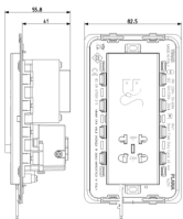
Zeichnung Dimensionen
