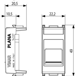
Zeichnung Dimensionen
