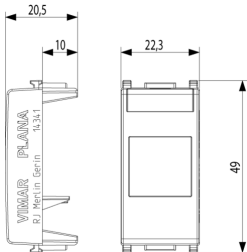
Zeichnung Dimensionen
