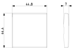
Zeichnung Dimensionen
