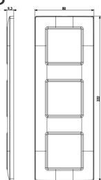
Zeichnung Dimensionen
