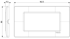
Zeichnung Dimensionen
