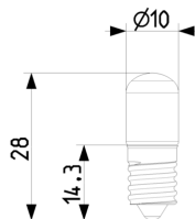
Zeichnung Dimensionen
