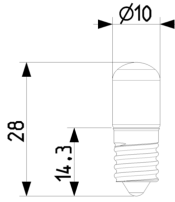
Zeichnung Dimensionen
