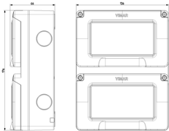
Zeichnung Dimensionen
