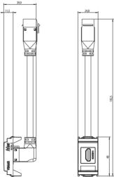
Zeichnung Dimensionen
