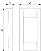
Zeichnung Dimensionen
