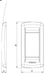
Zeichnung Dimensionen
