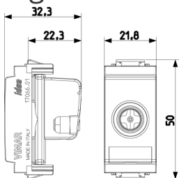
Zeichnung Dimensionen
