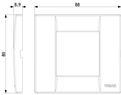
Zeichnung Dimensionen
