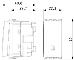
Zeichnung Dimensionen
