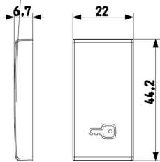
Zeichnung Dimensionen
