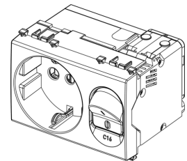
3D-Ansicht
