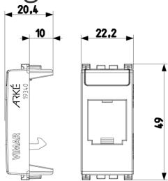
Zeichnung Dimensionen
