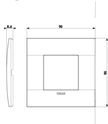
Zeichnung Dimensionen
