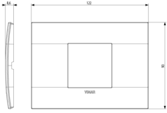
Zeichnung Dimensionen
