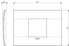
Zeichnung Dimensionen
