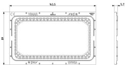
Zeichnung Dimensionen
