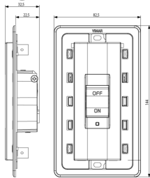
Zeichnung Dimensionen
