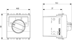
Zeichnung Dimensionen
