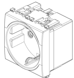
3D-Ansicht
