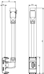
Zeichnung Dimensionen
