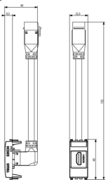
Zeichnung Dimensionen
