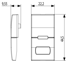
Zeichnung Dimensionen
