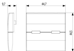
Zeichnung Dimensionen
