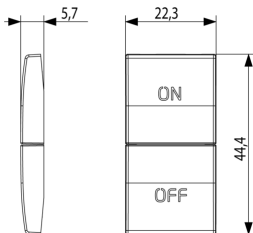
Zeichnung Dimensionen
