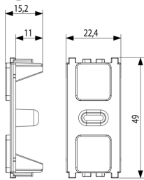
Zeichnung Dimensionen
