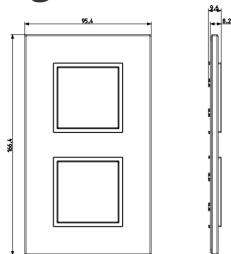
Zeichnung Dimensionen
