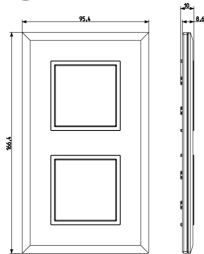
Zeichnung Dimensionen
