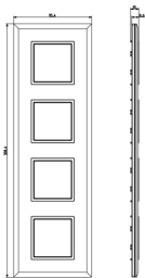
Zeichnung Dimensionen
