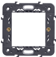
21602 - Rahmen 2M +Kralle Abst71mm
