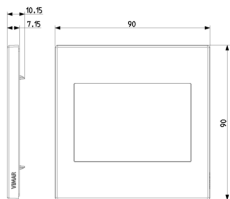
Zeichnung Dimensionen
